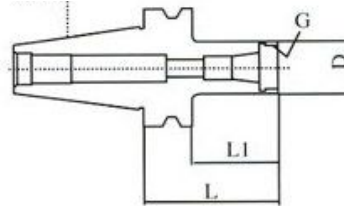
■ 7/24テーパ
